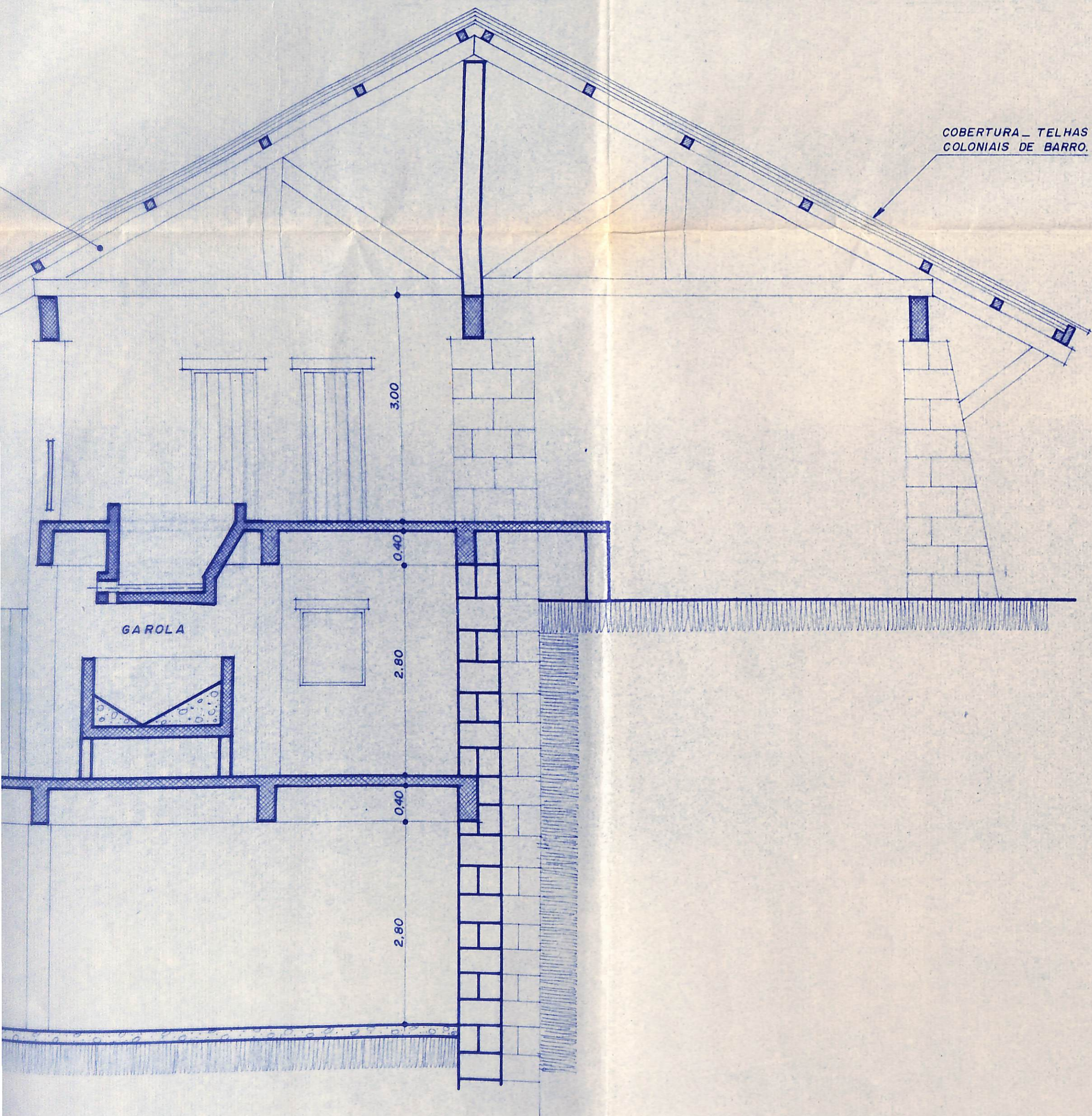
CORTE TRANSVERSAL - RECEBIMENTO E ELABORAÇÃO ESCALA 1:50
